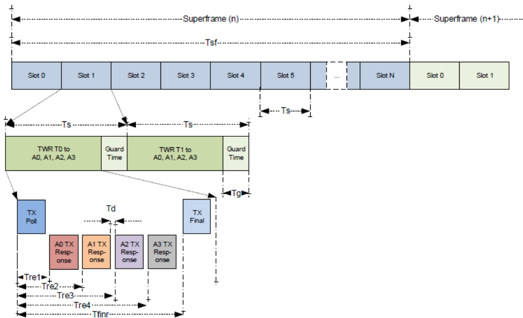
图 5-1 SLOT 分配
